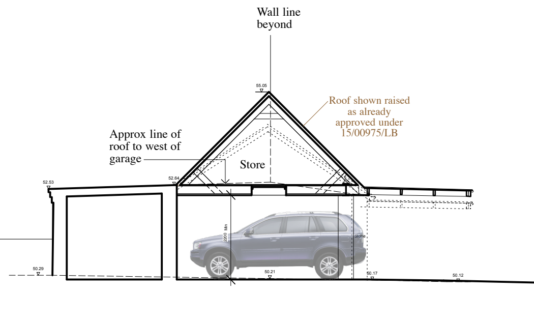
Elevation BB
