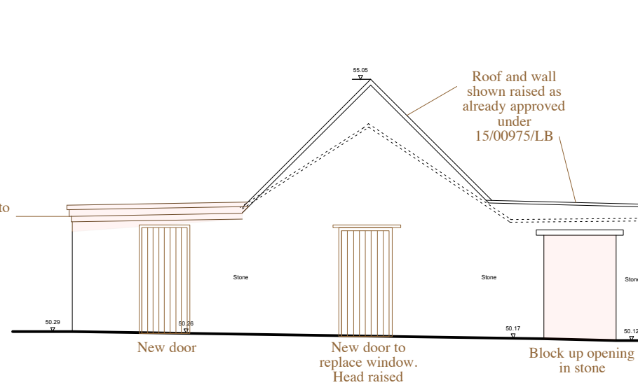
Elevation BB
