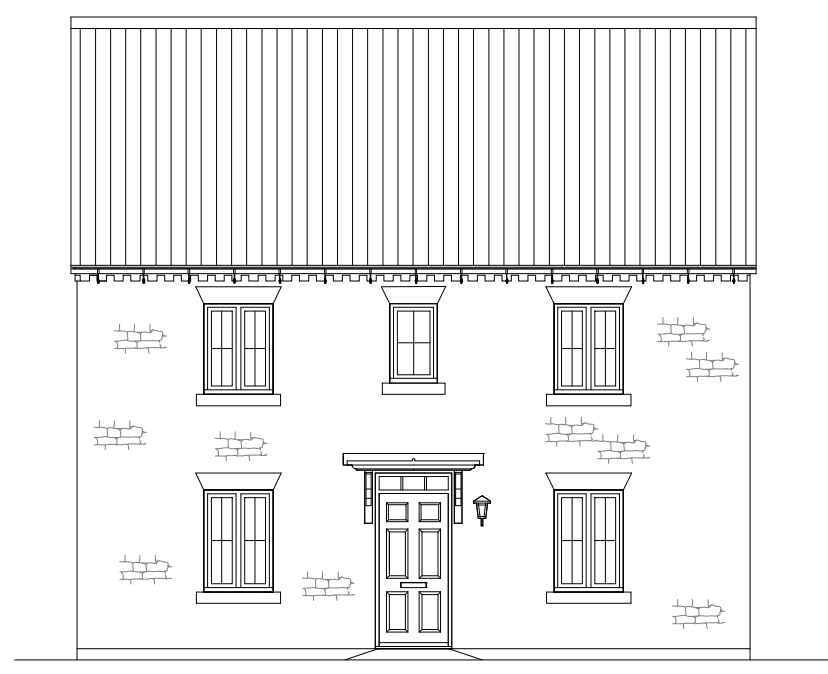
MOR FRONT ELEVATION 2
