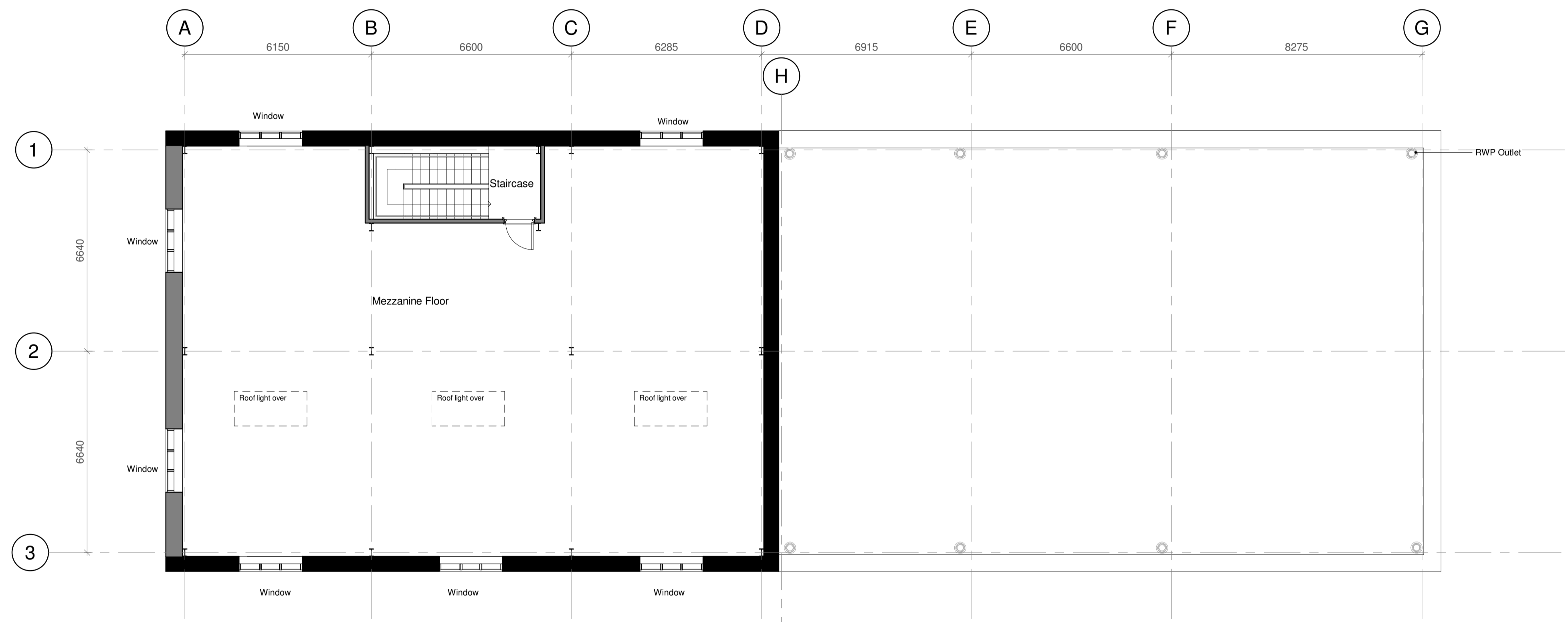
Mezzanine Plan 1 : 100
