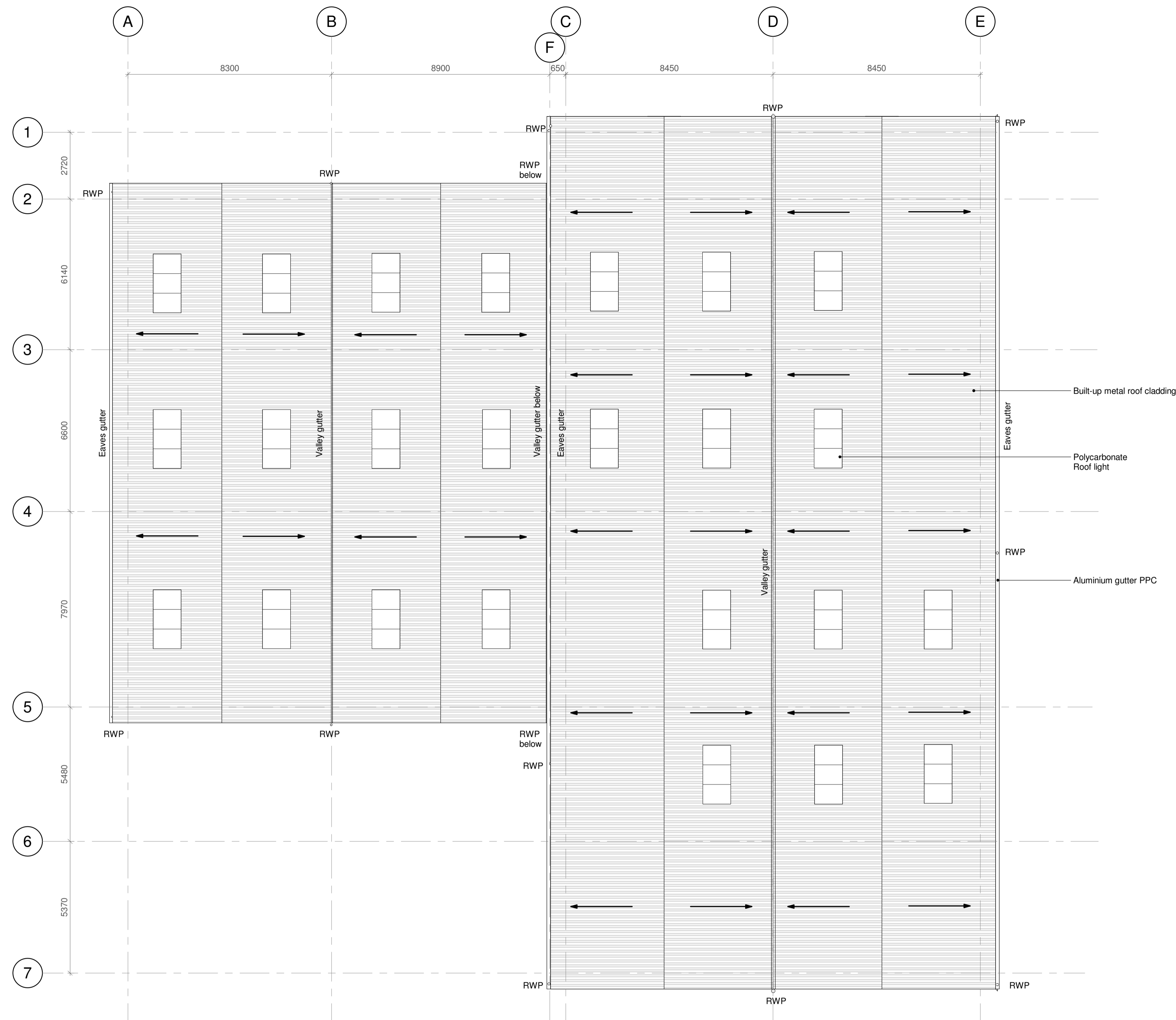
Roof Plan 1 : 100
