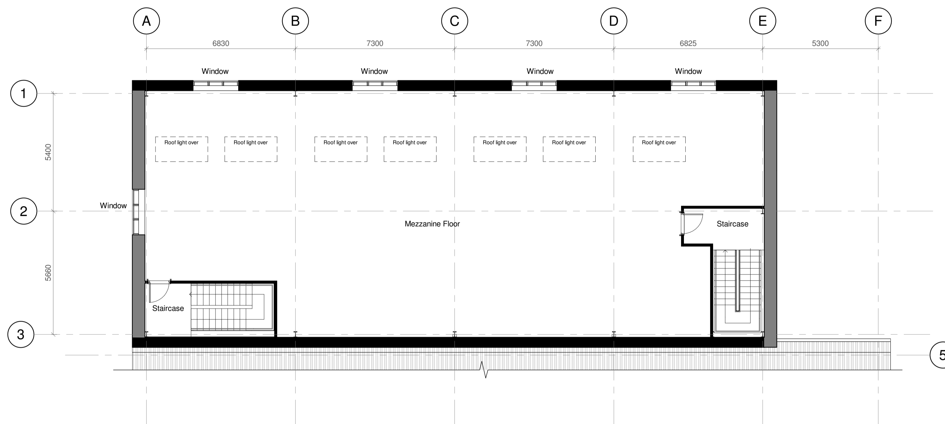
Mezzanine Plan 1 : 100
