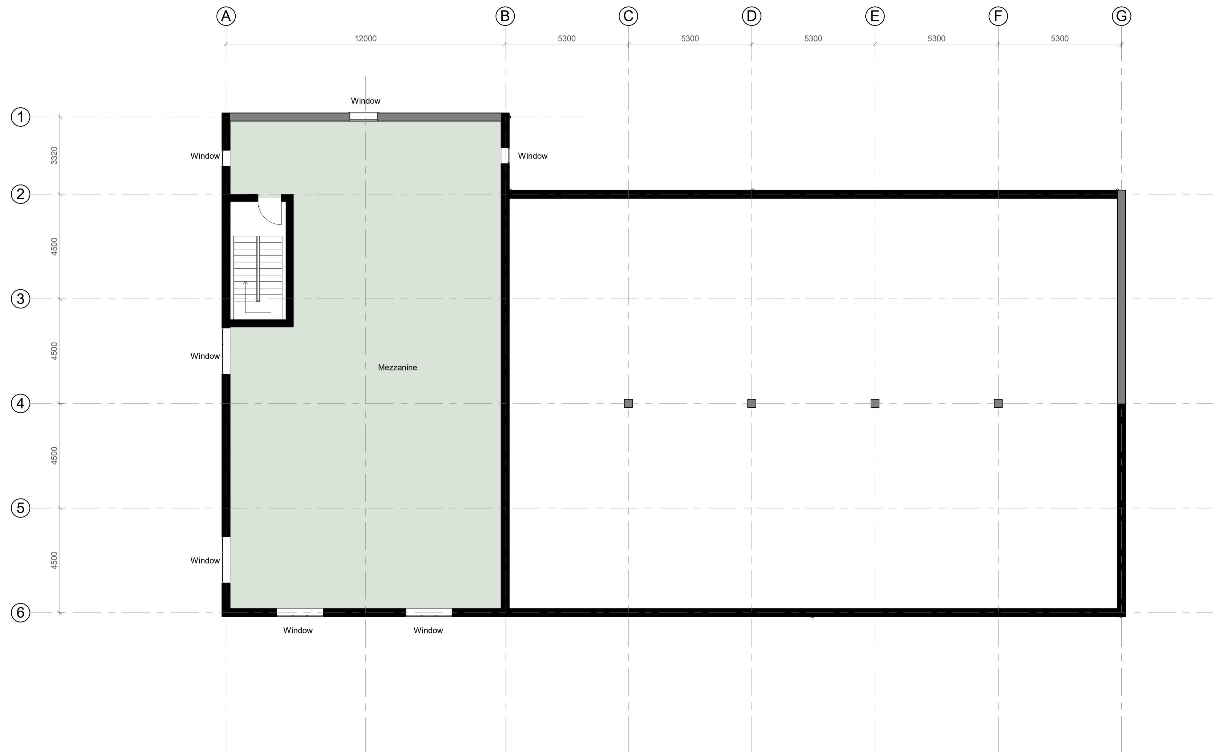
Mezzanine Plan 1 : 100
