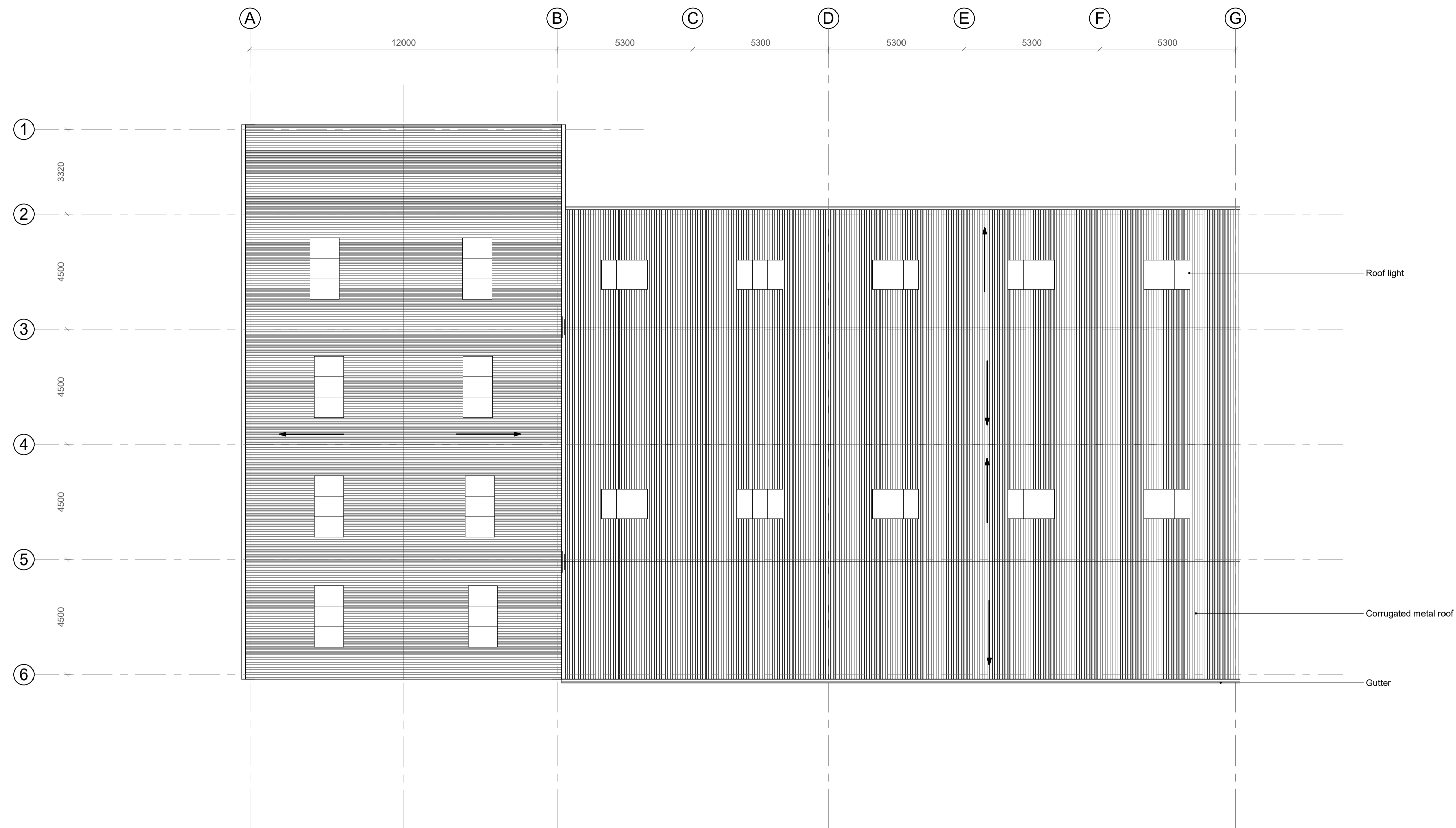
Roof Plan 1 : 100
