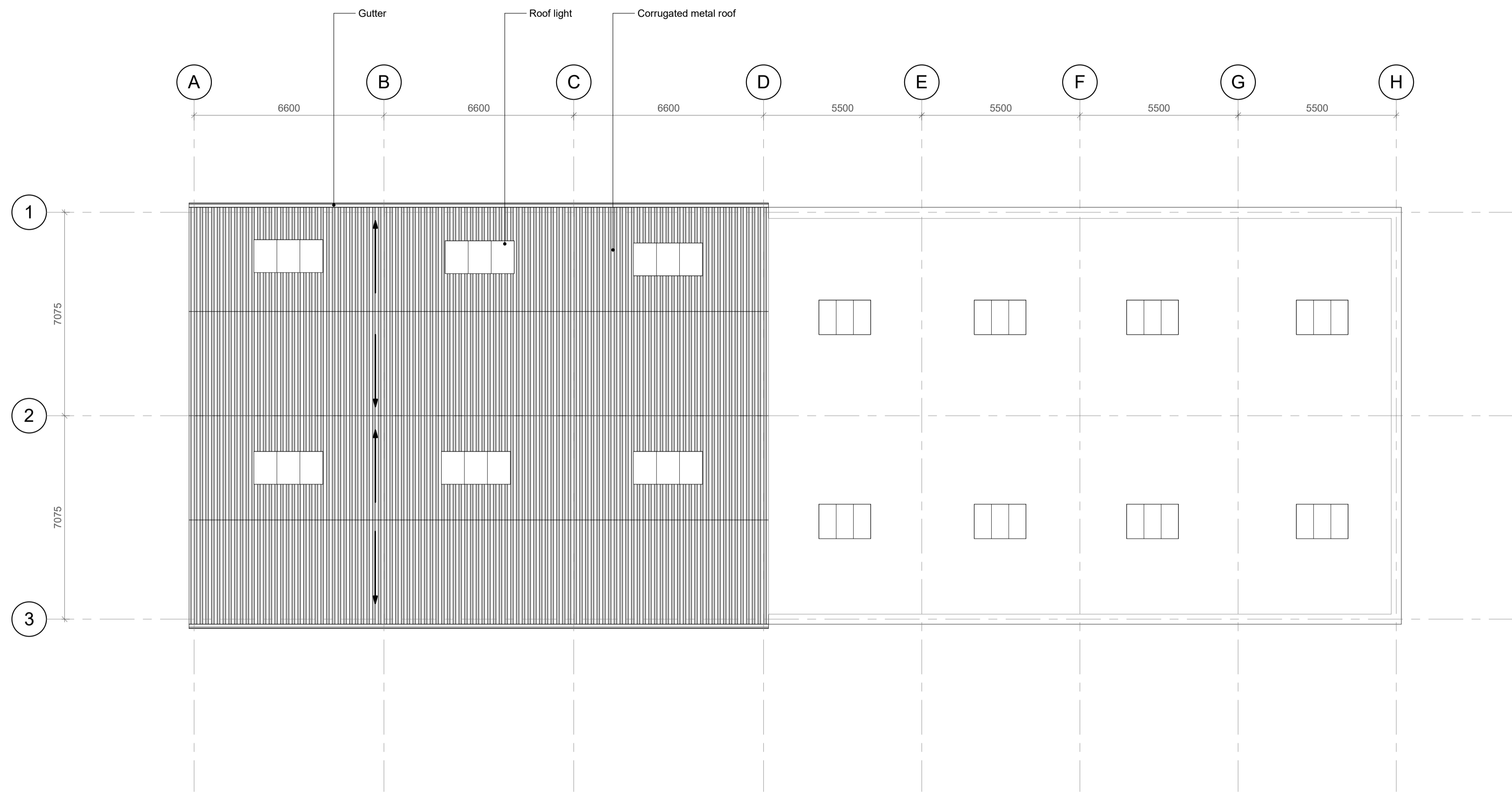
Roof Plan 1 : 100
