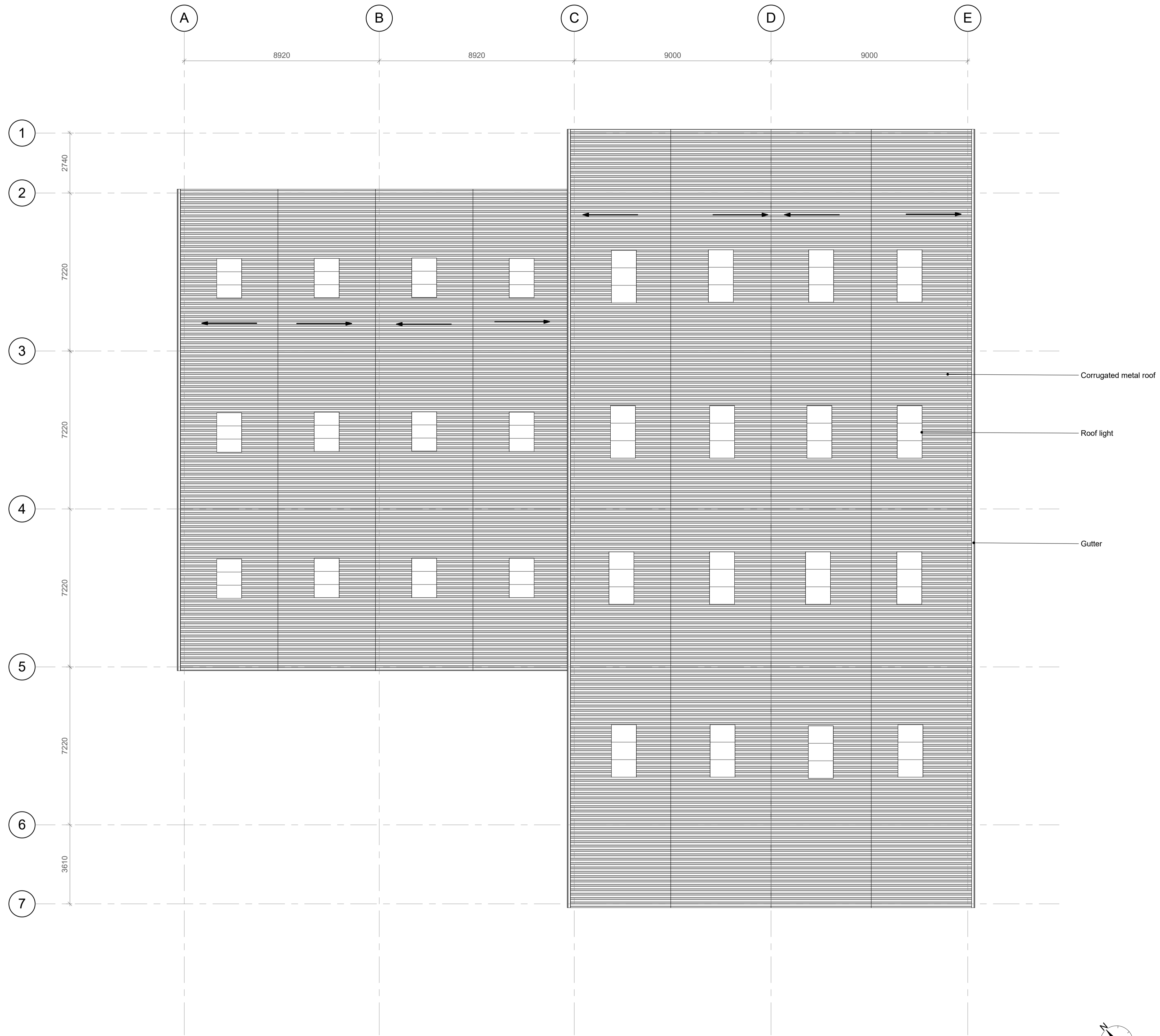
Roof Plan 1 : 100
