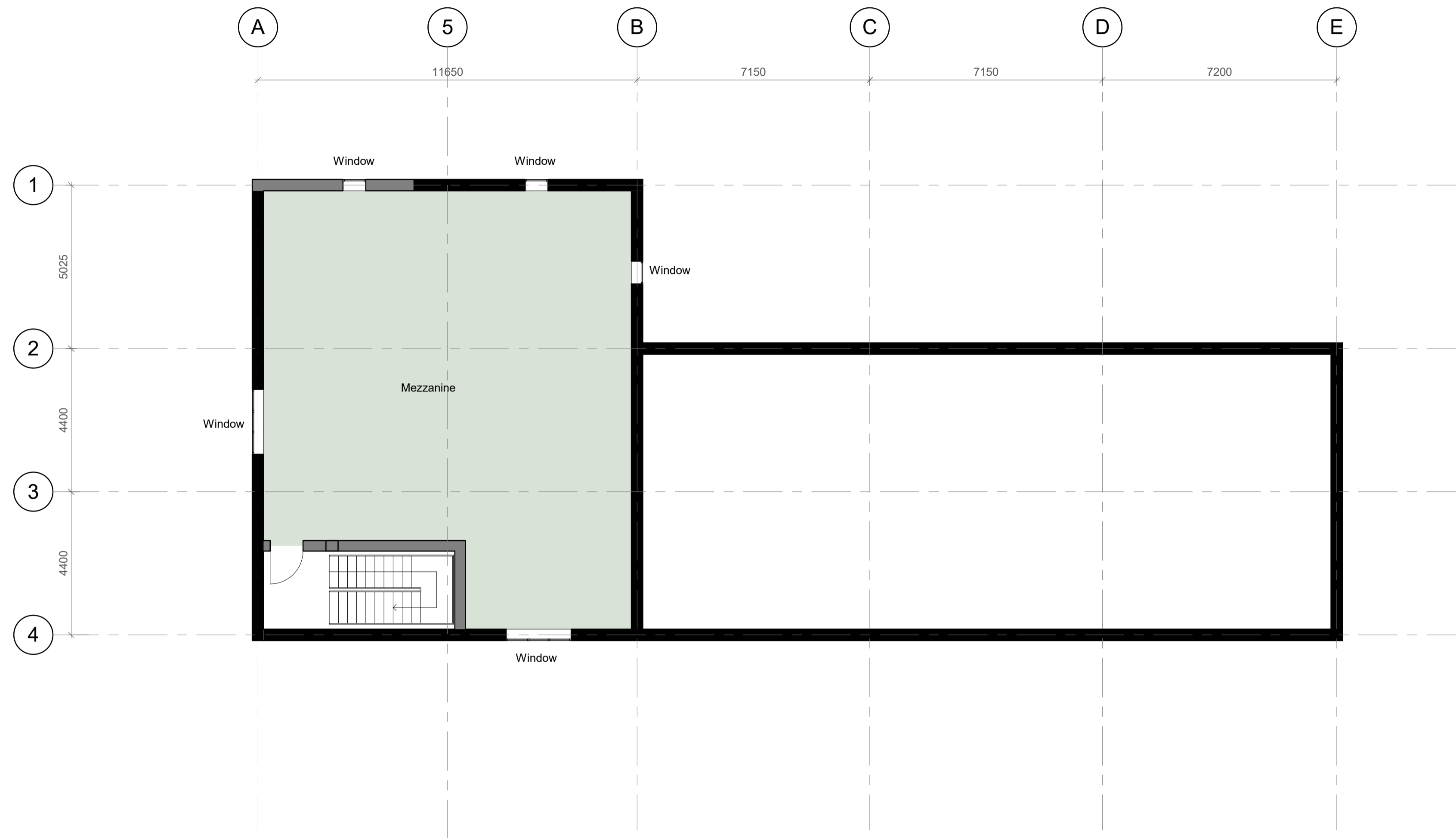
Mezzanine Plan 1 : 100
