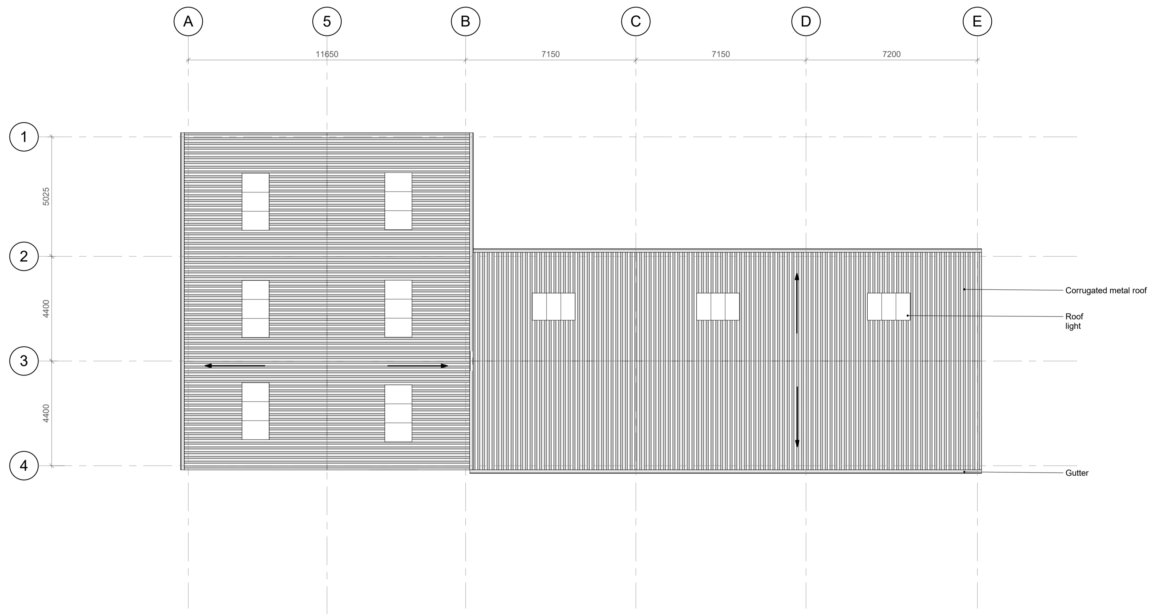
Roof Plan 1 : 100
