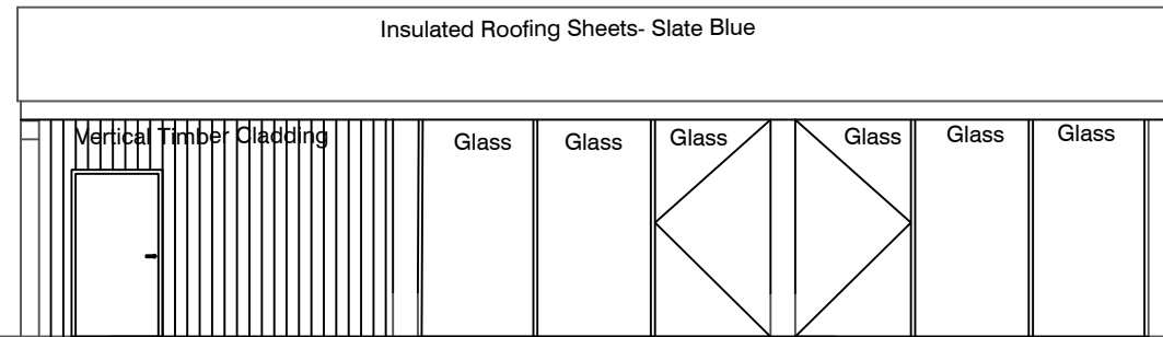
Elevation 1
