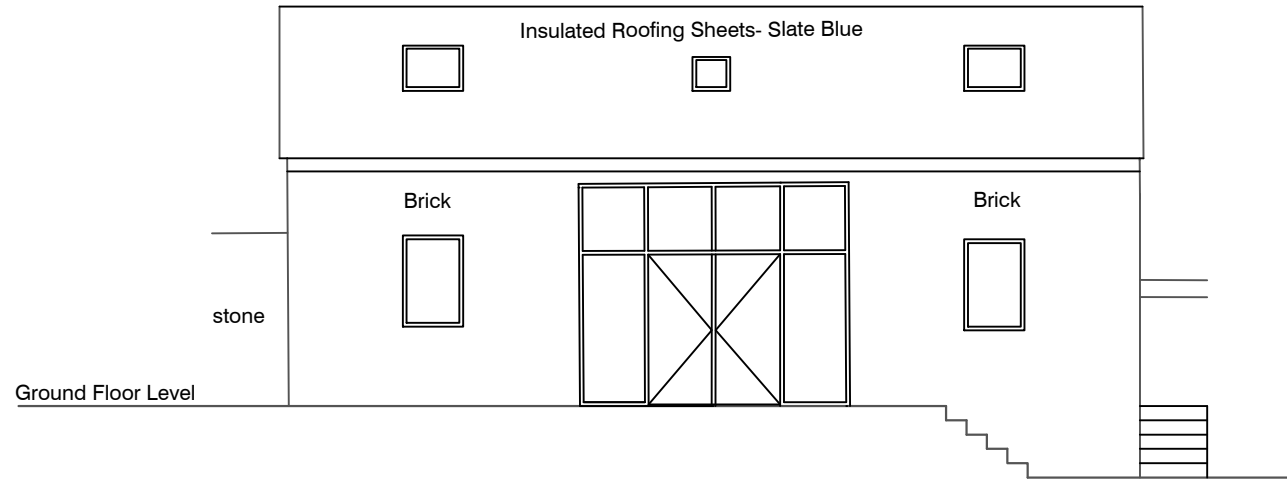
Elevation 1
