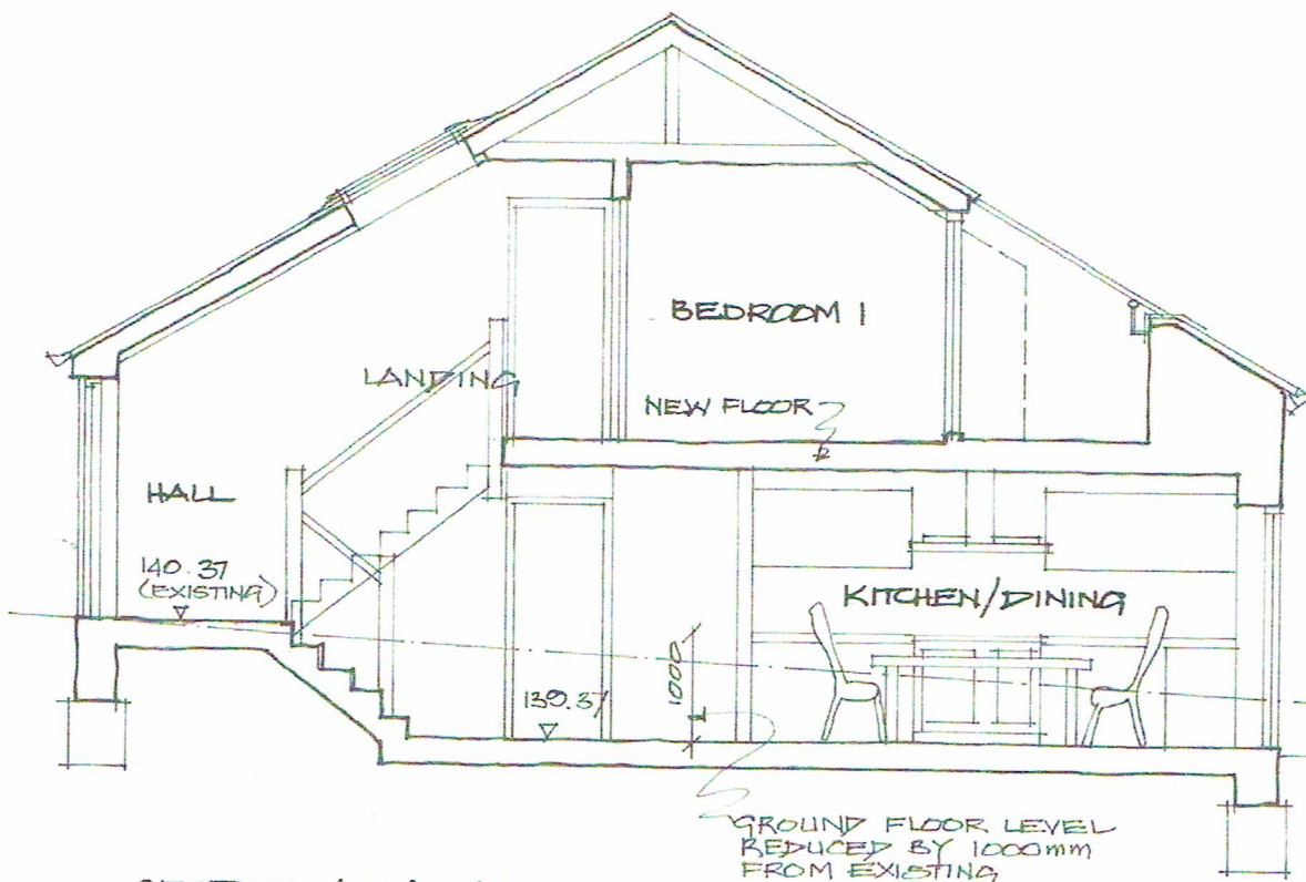
SECTION A-A 1:50
