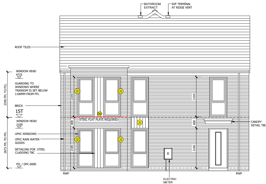
SIDE ELEVATION PLOTS 361-364
