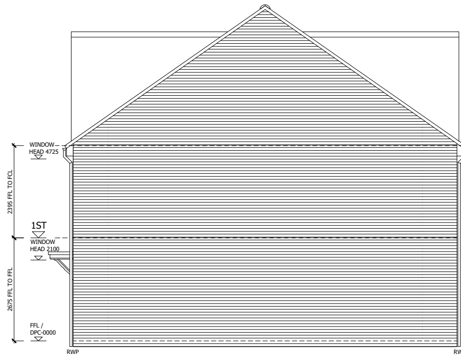
SIDE ELEVATION PLOTS 361-364
