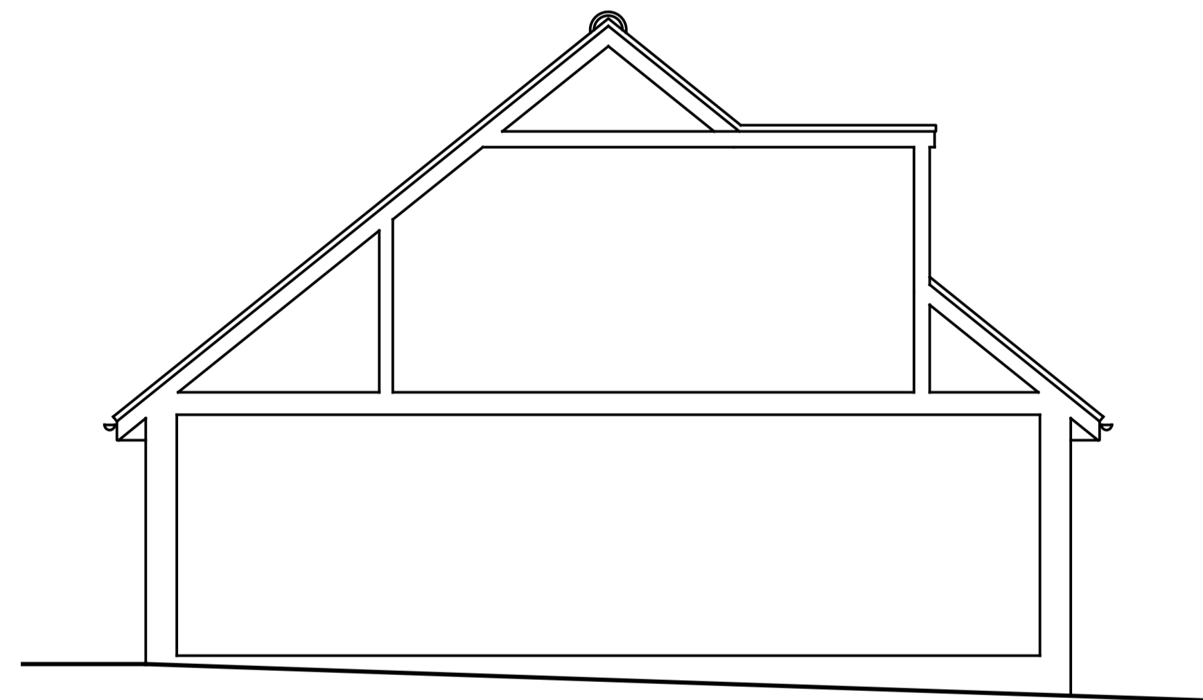
Cross Section Scale 1:50 0.0m 1.0m 2.0m 3.0m 4.0m 5.0m
