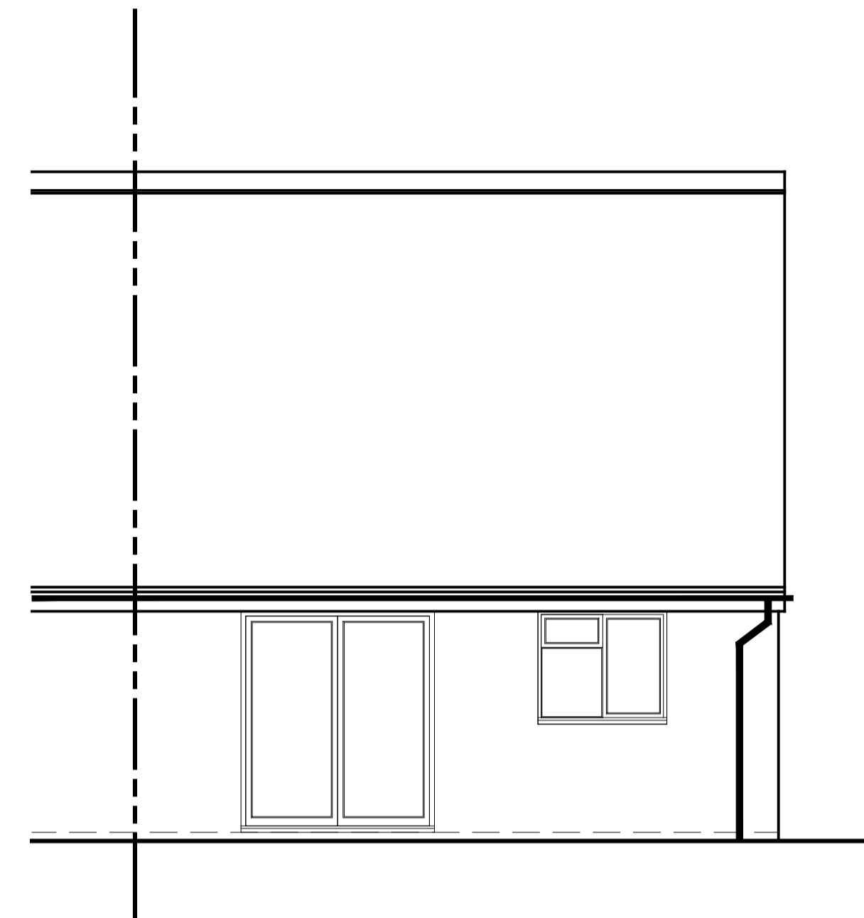
North Elevation Scale 1:50 0.0m 1.0m 2.0m 3.0m 4.0m 5.0m
