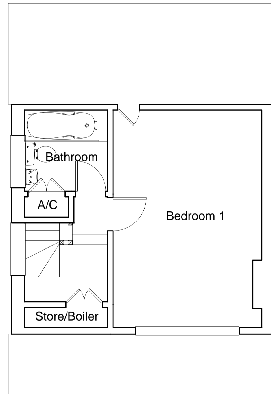
First Floor Plan Scale 1:50 0.0m 1.0m 2.0m 3.0m 4.0m 5.0m
