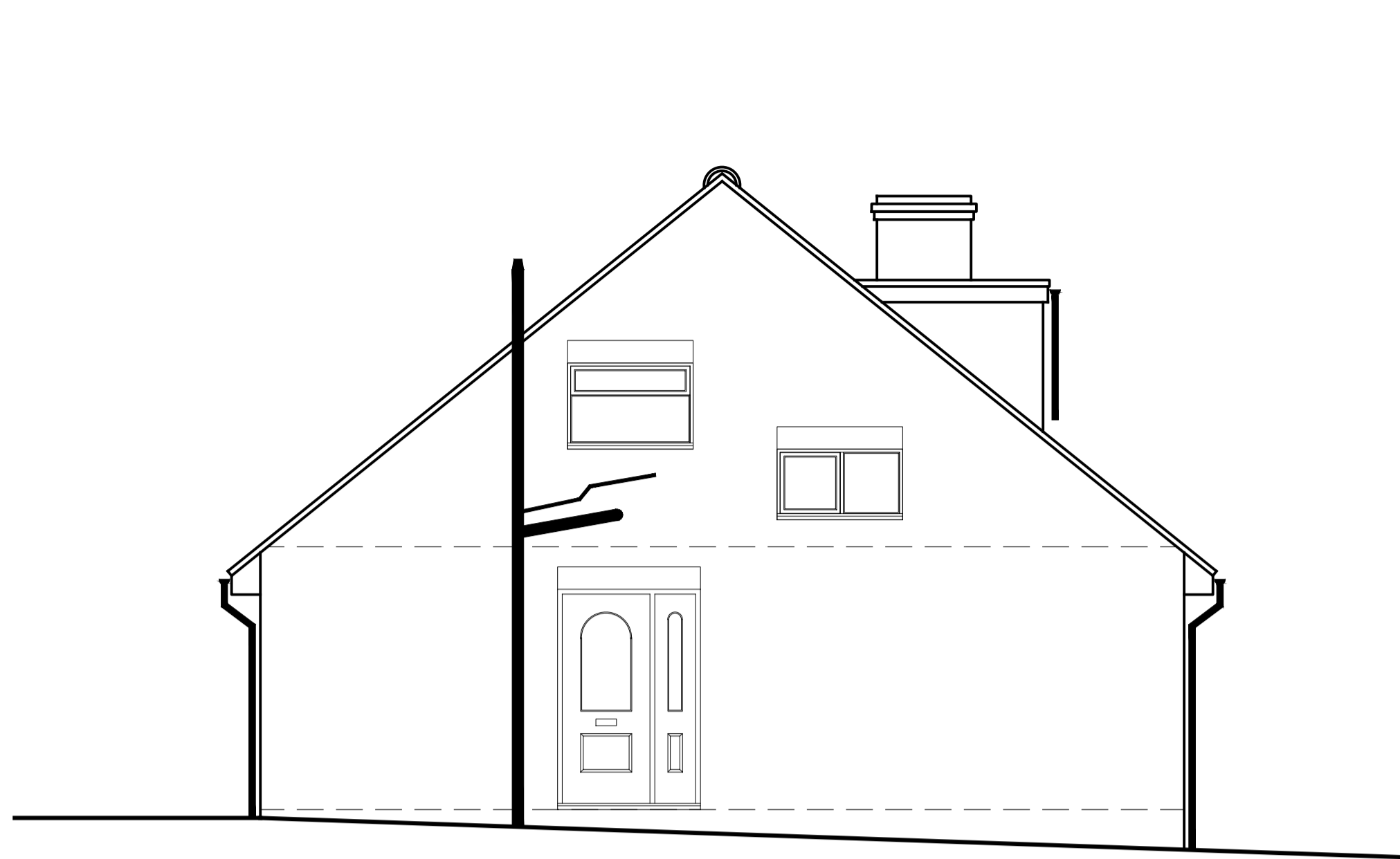
West Elevation Scale 1:50 0.0m 1.0m 2.0m 3.0m 4.0m 5.0m
