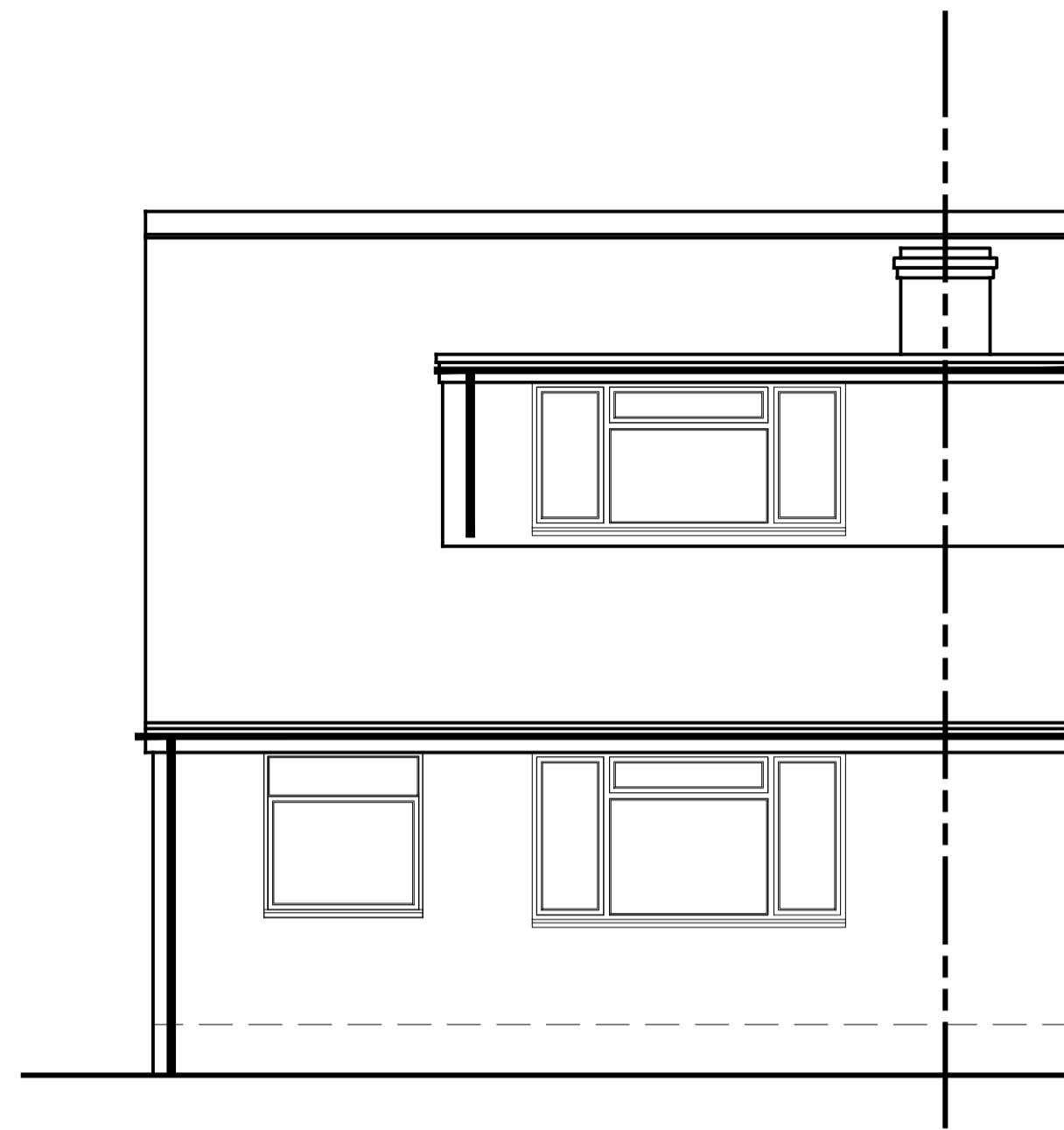
South Elevation Scale 1:50 0.0m 1.0m 2.0m 3.0m 4.0m 5.0m
