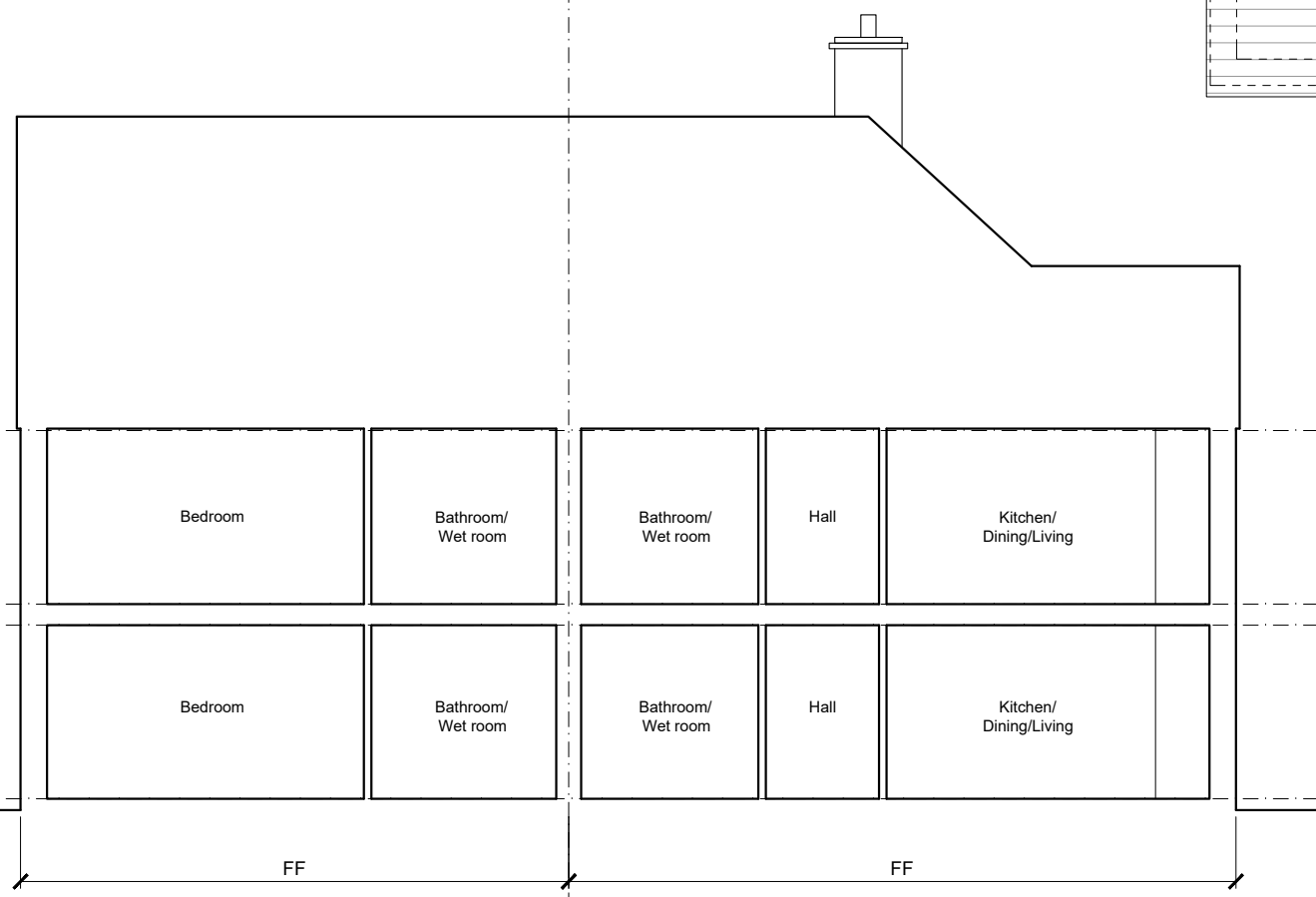
Section HH - 6xF 1:100 (A3)
