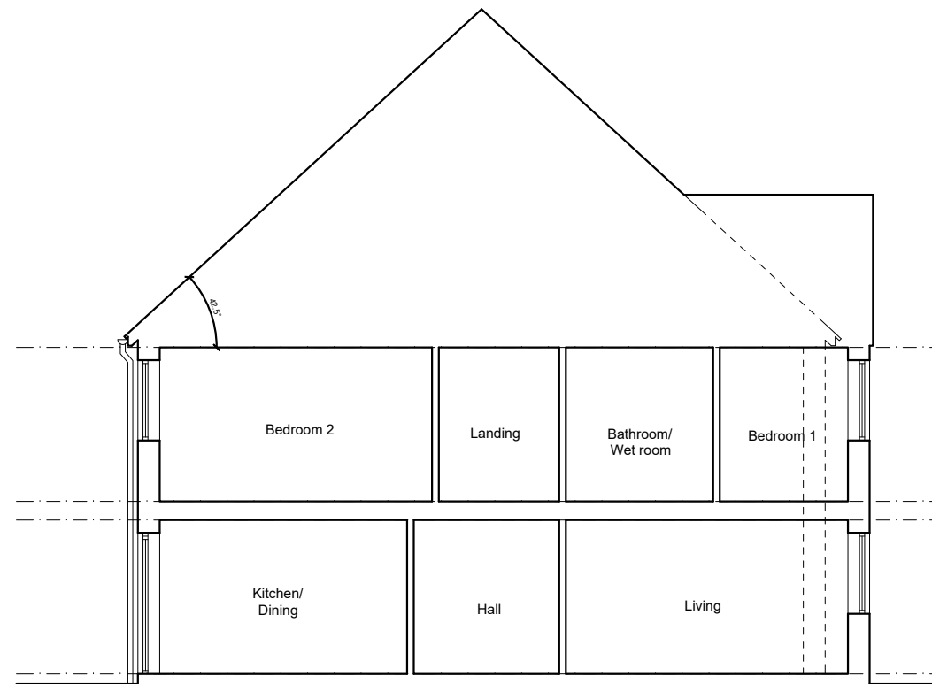
Section DD 1:100 (A3)
