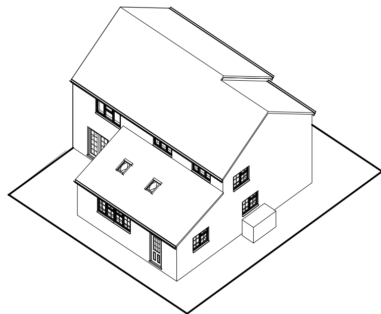
3 9001 AXO 03 - EXISTING
