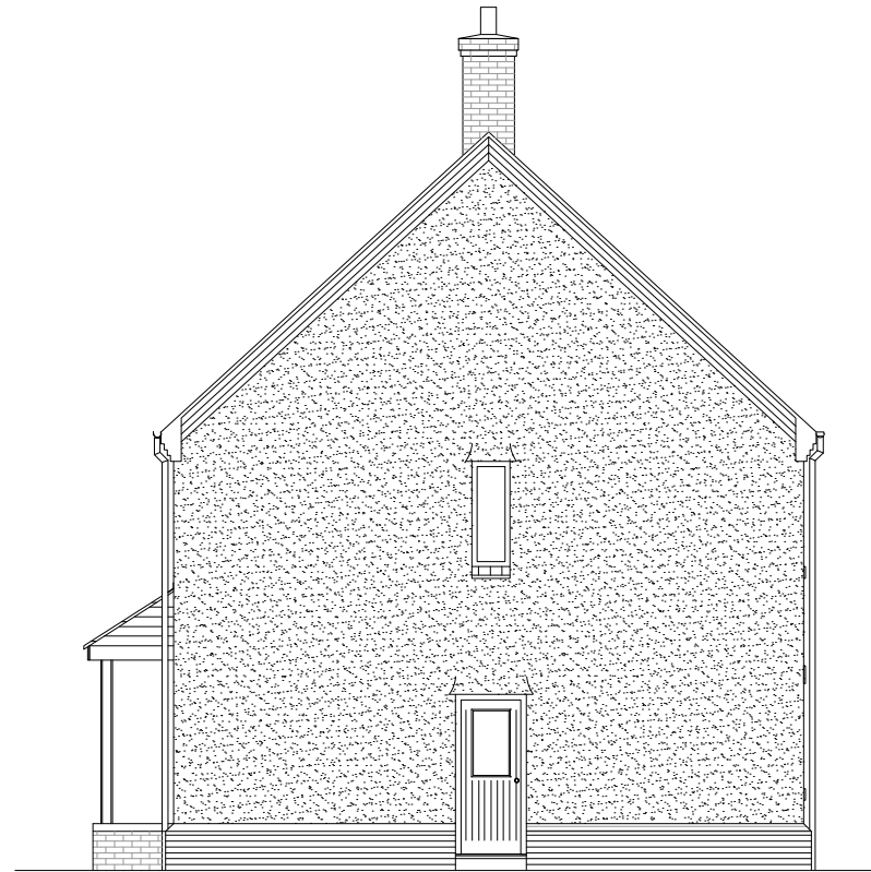
RIGHT ELEVATION
