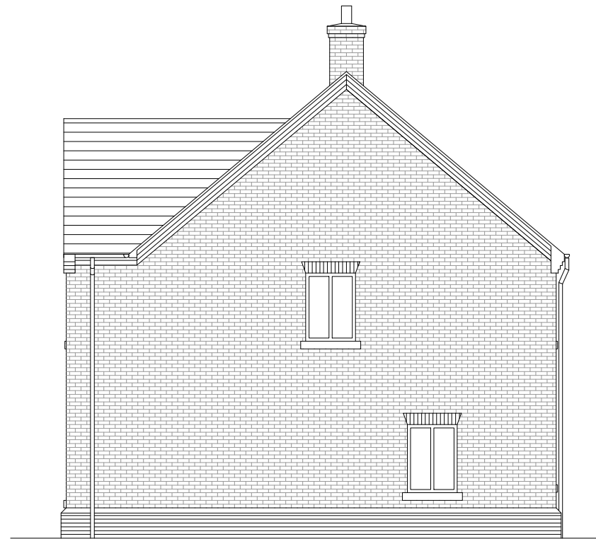
RIGHT ELEVATION
