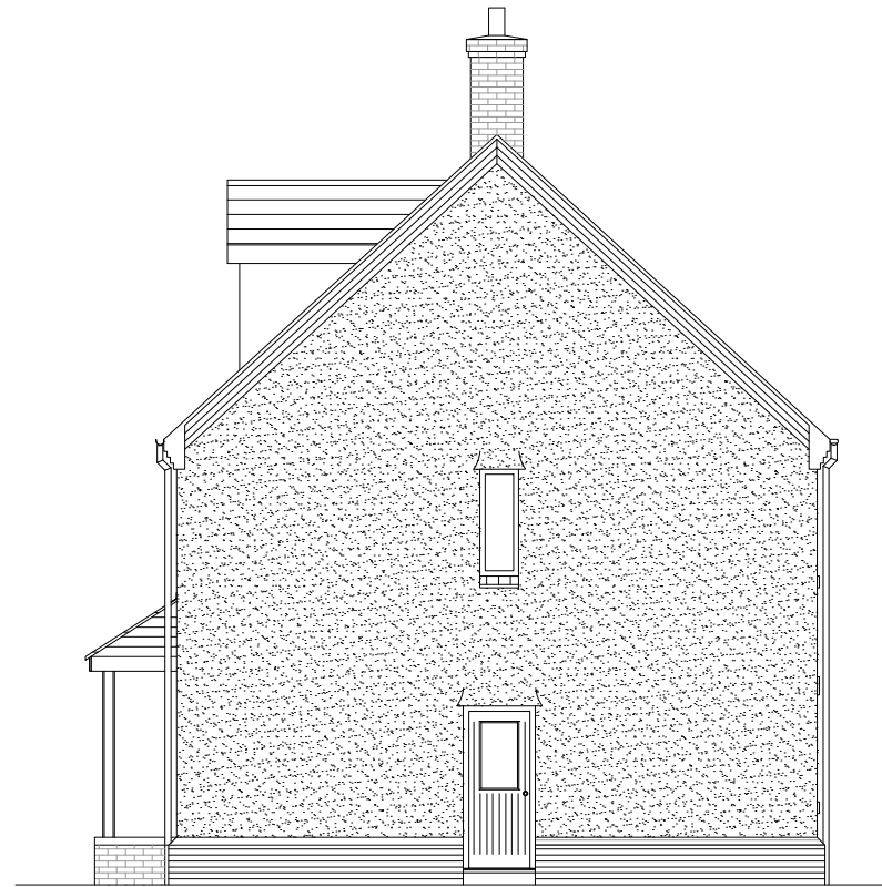
RIGHT ELEVATION
