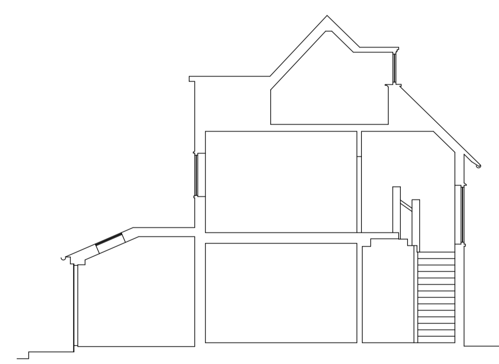
Datum 105.00m SECTION A-A
