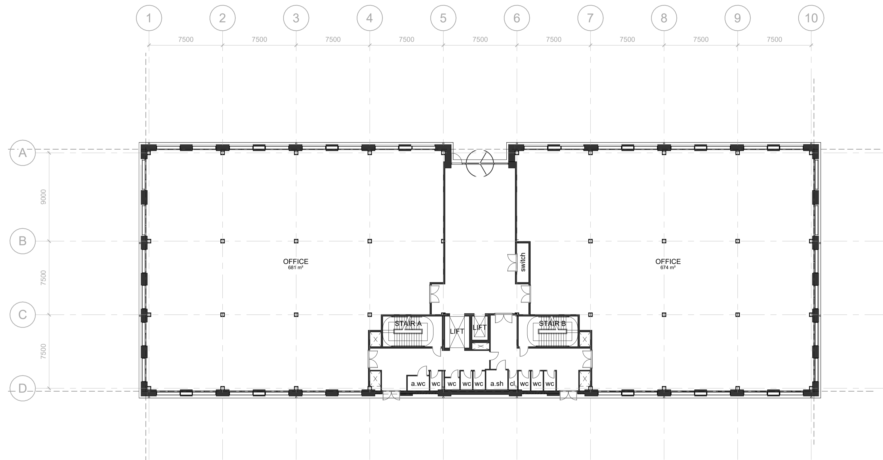
Level 00 1 : 200
