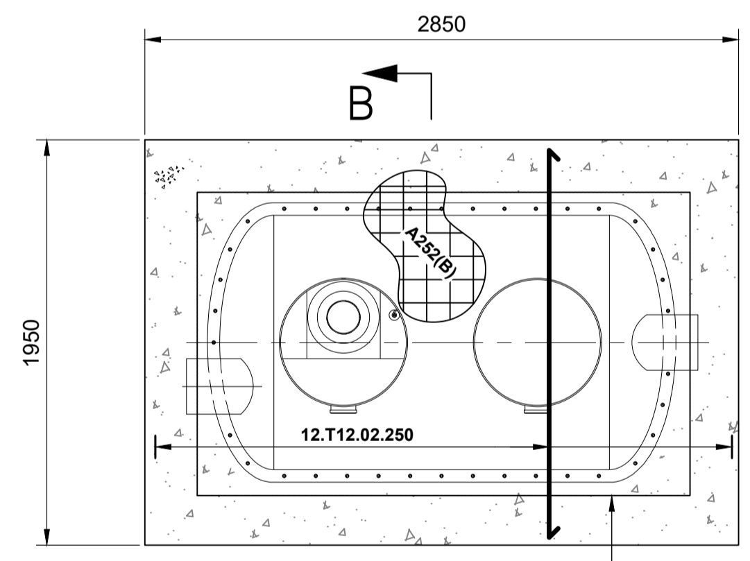
TOP PLAN 1:25
