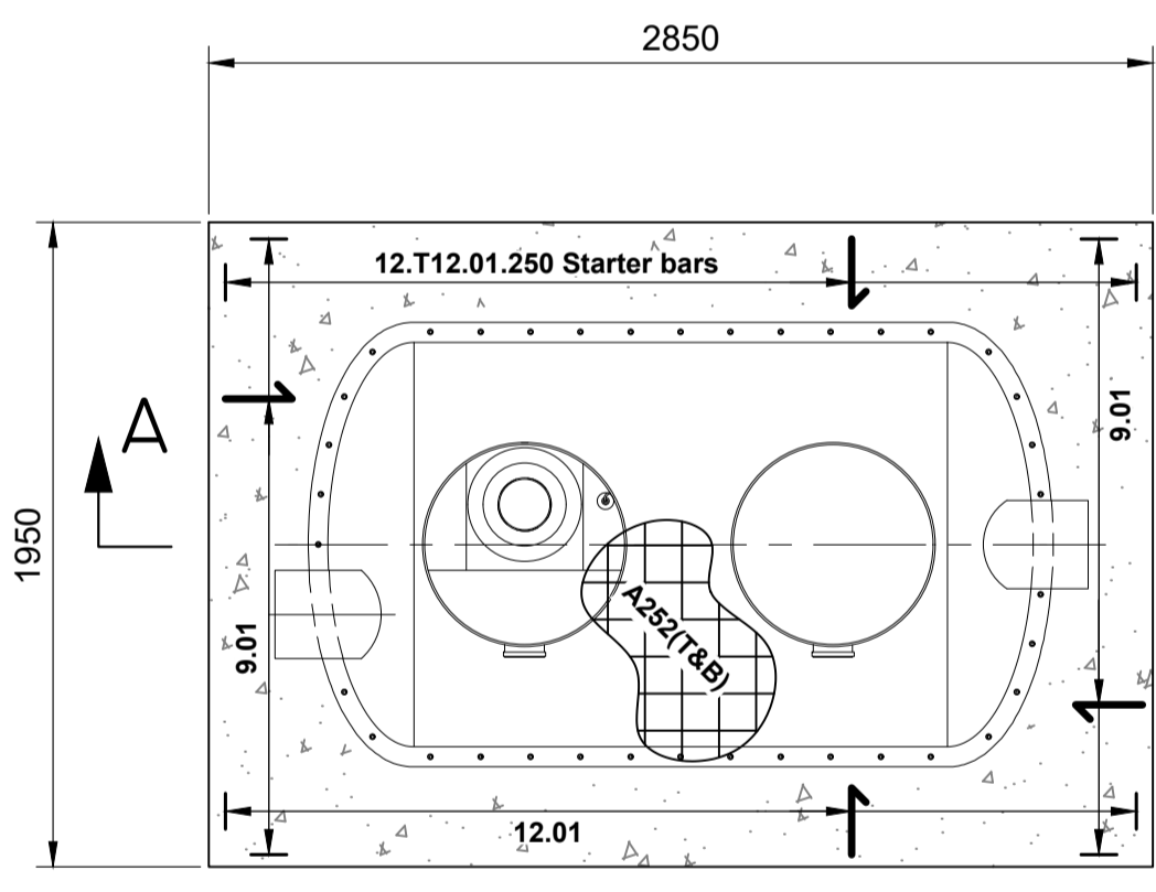
BASE PLAN 1:25
