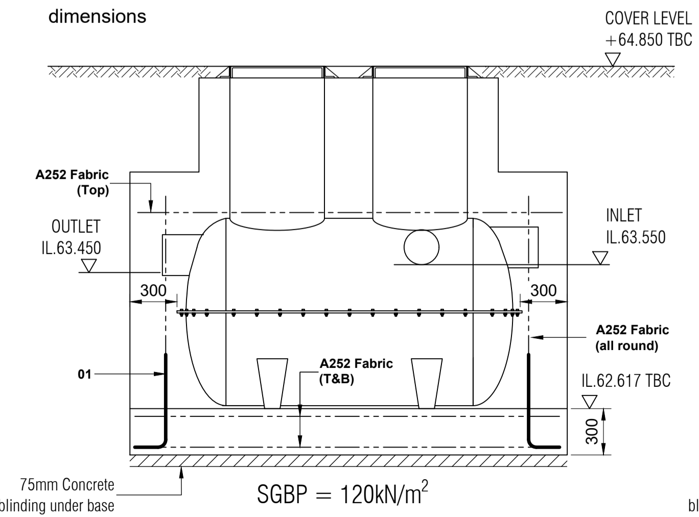
SECTION A-A 1:25
