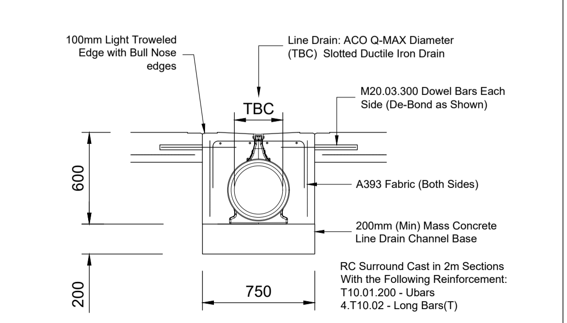
ACO Qmax Detail 1:25
