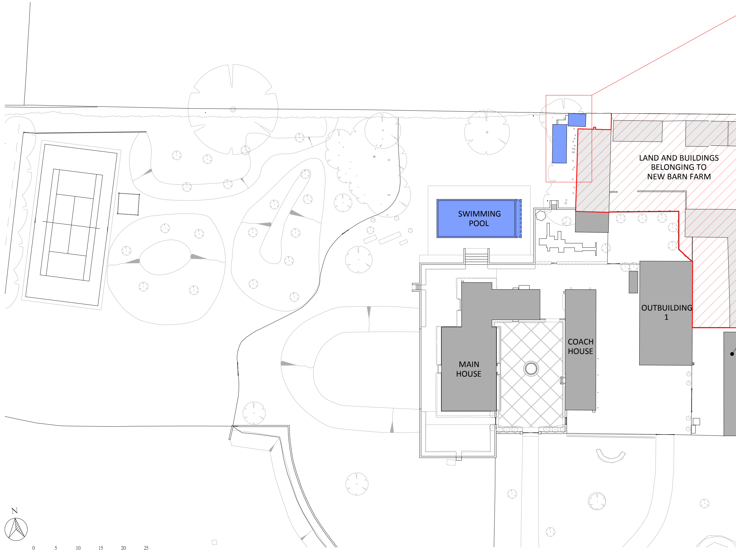
Site Plan 1:500
