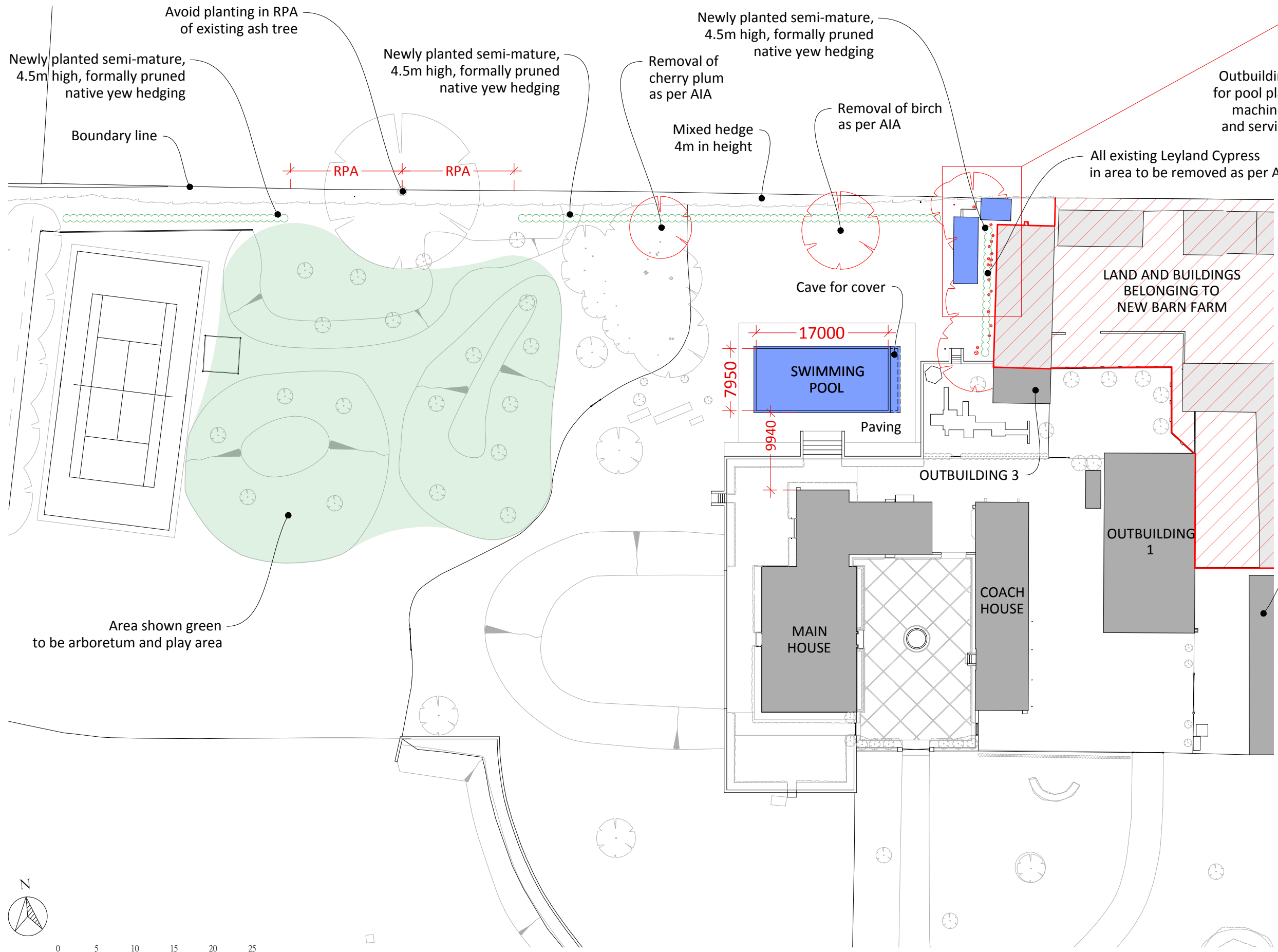
Site Plan 1:500
