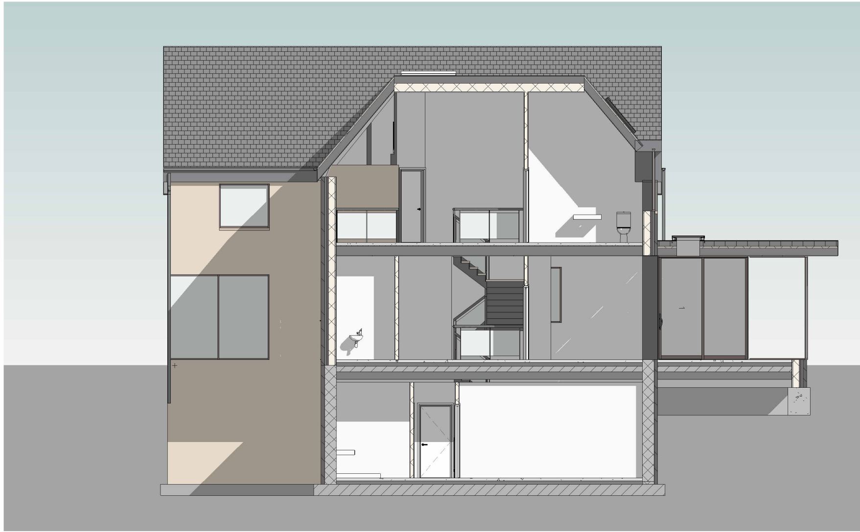
Section AA 1 : 100
