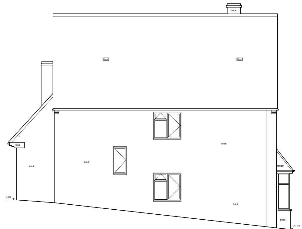
4 Existing West Elevation Scale: 1:100
