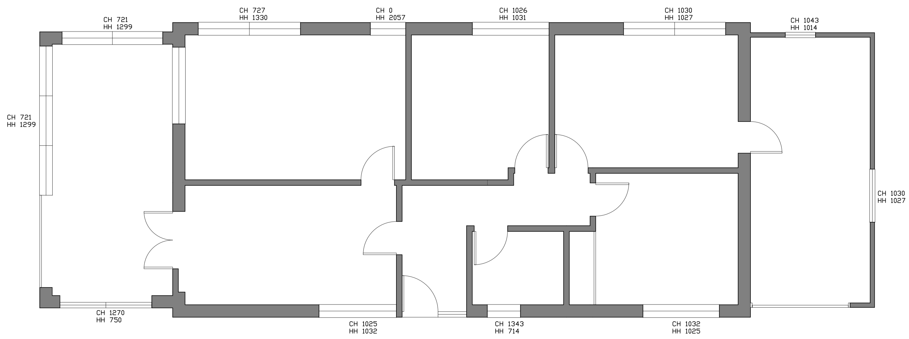
Ground Floor Plan Scale 1:50 0.0m 1.0m 2.0m 3.0m 4.0m 5.0m
