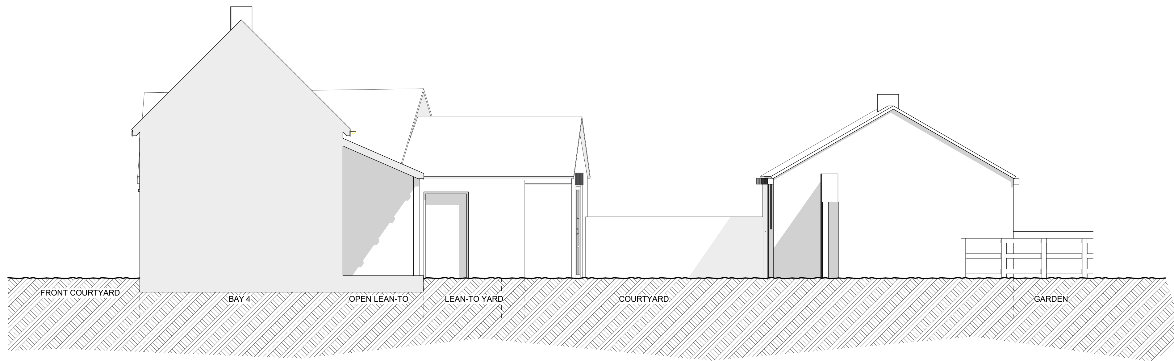
C-C EXISTING ELEVATIONS 202 Scale: 1:50 @ A1 / 1:100 @ A3
