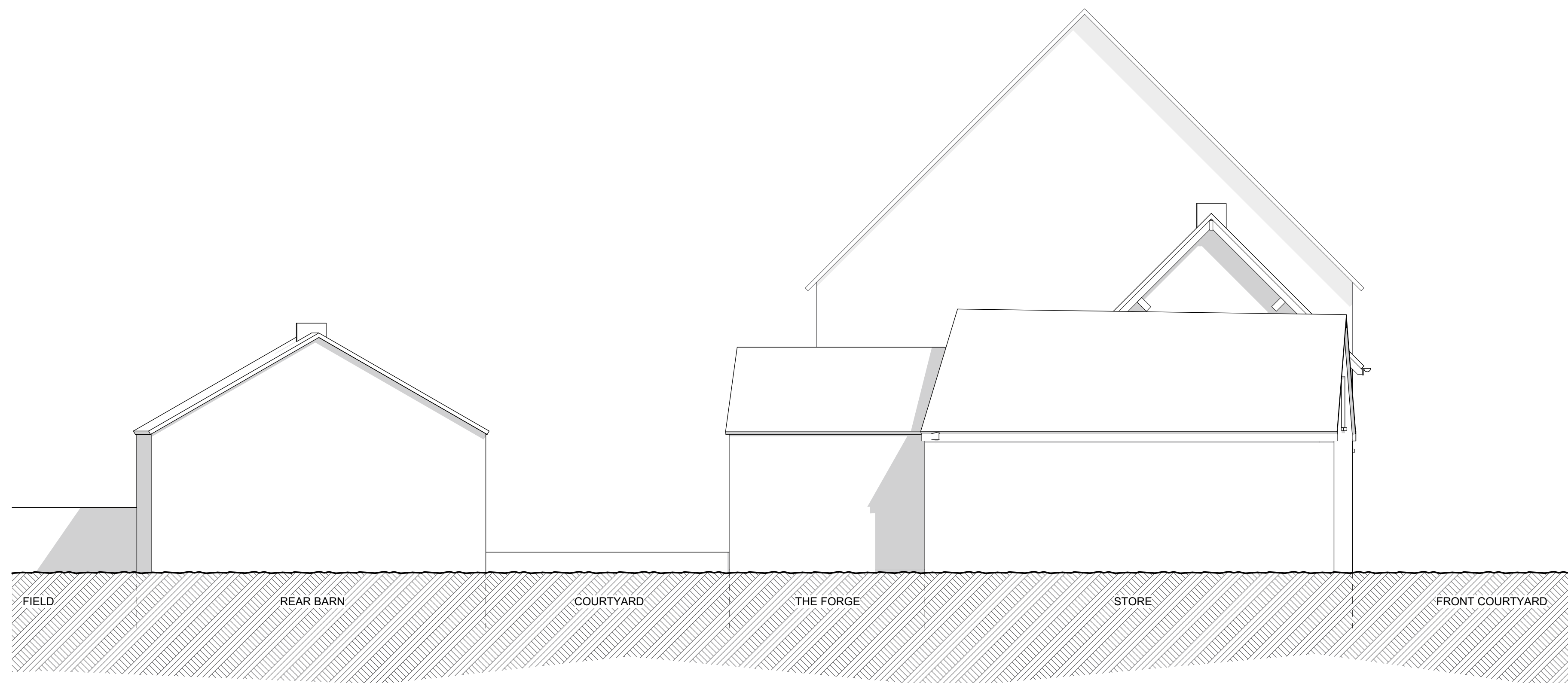
D-D EXISTING ELEVATIONS 202 Scale: 1:50 @ A1 / 1:100 @ A3
