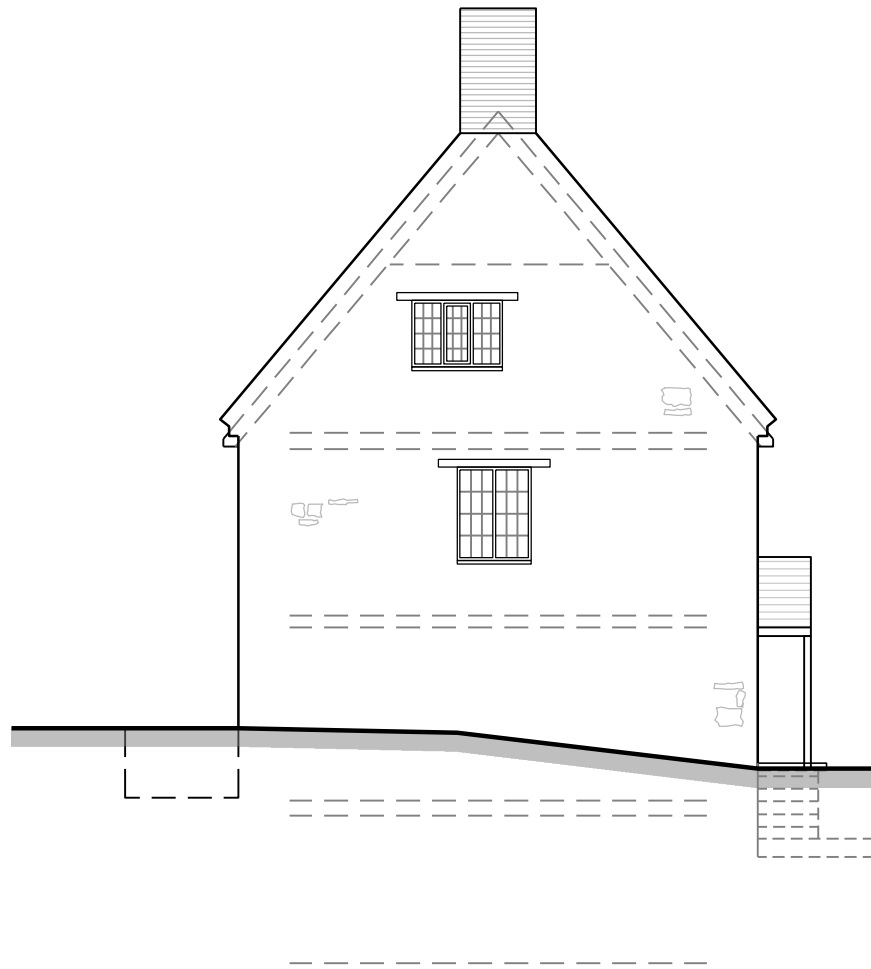
Existing West Elevation Scale: 1:100
