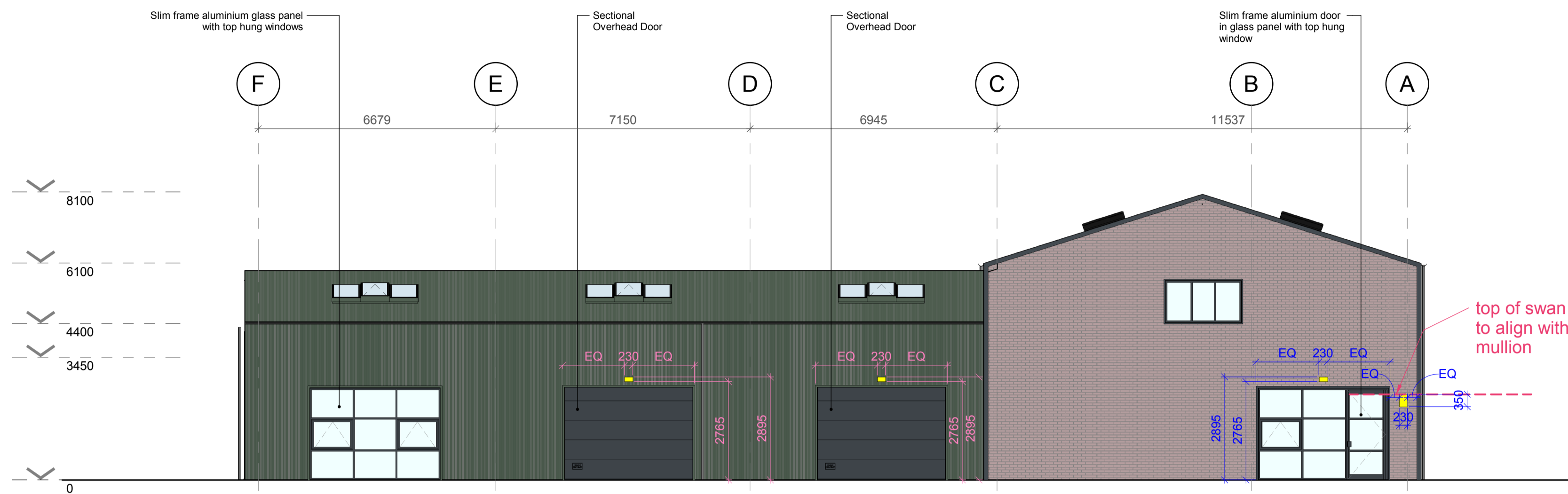
1. NE Elevation 1 : 100
