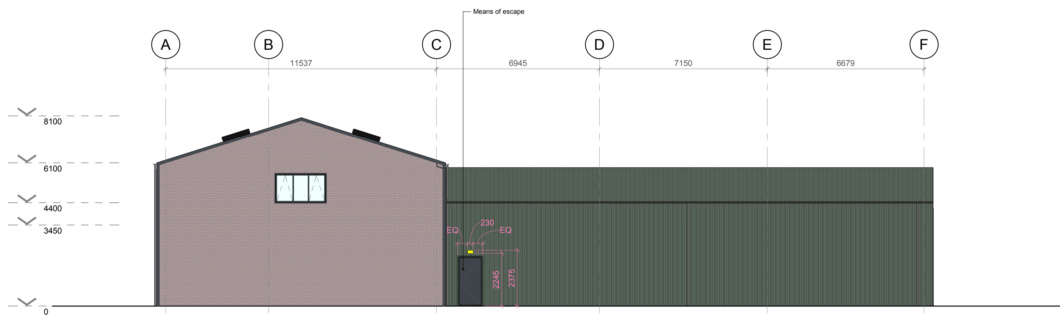
3. SW Elevation 1 : 100
