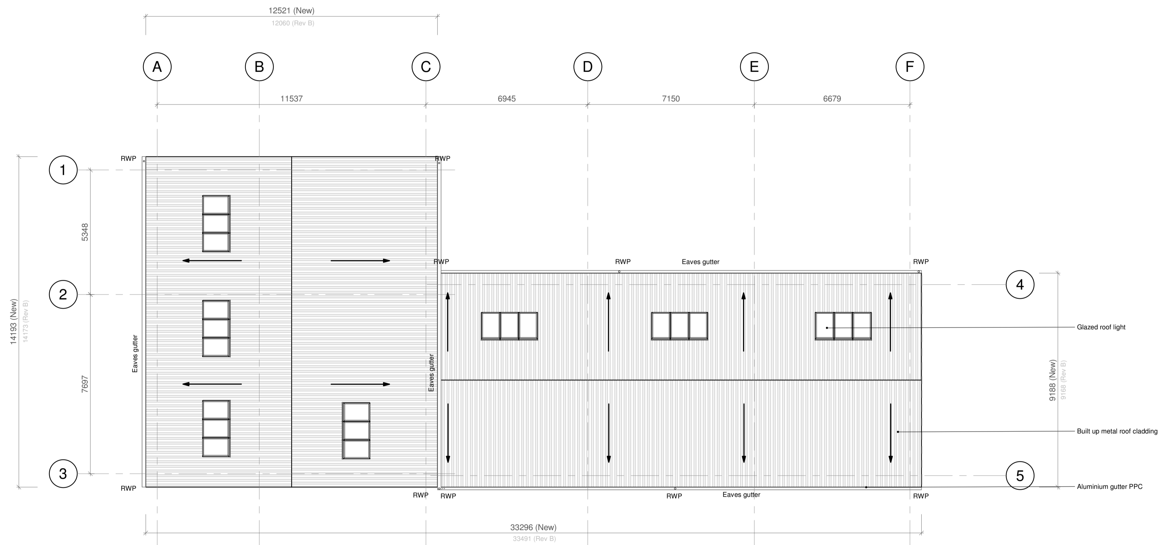
Roof Plan 1 : 100
