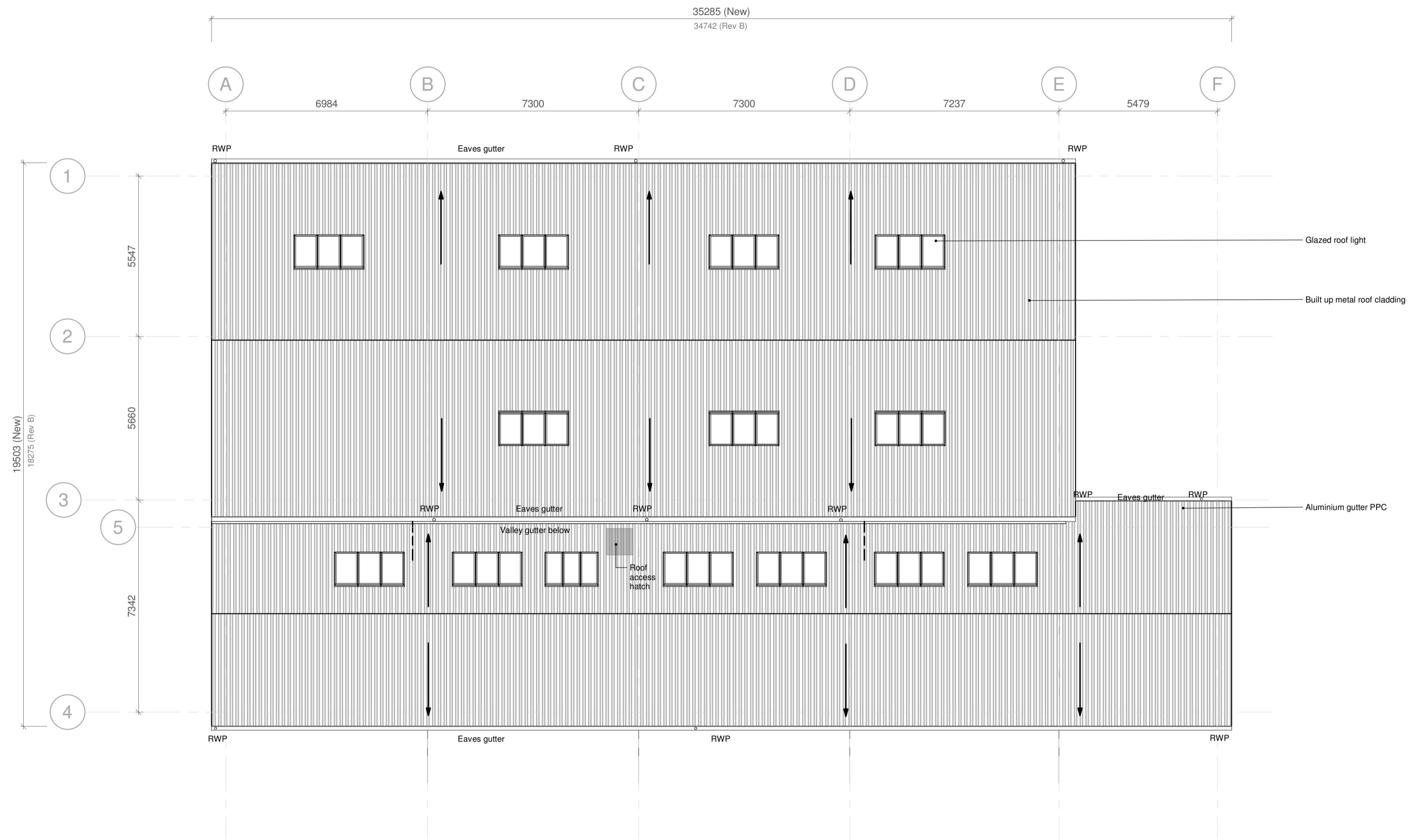
Roof Plan 1 : 100
