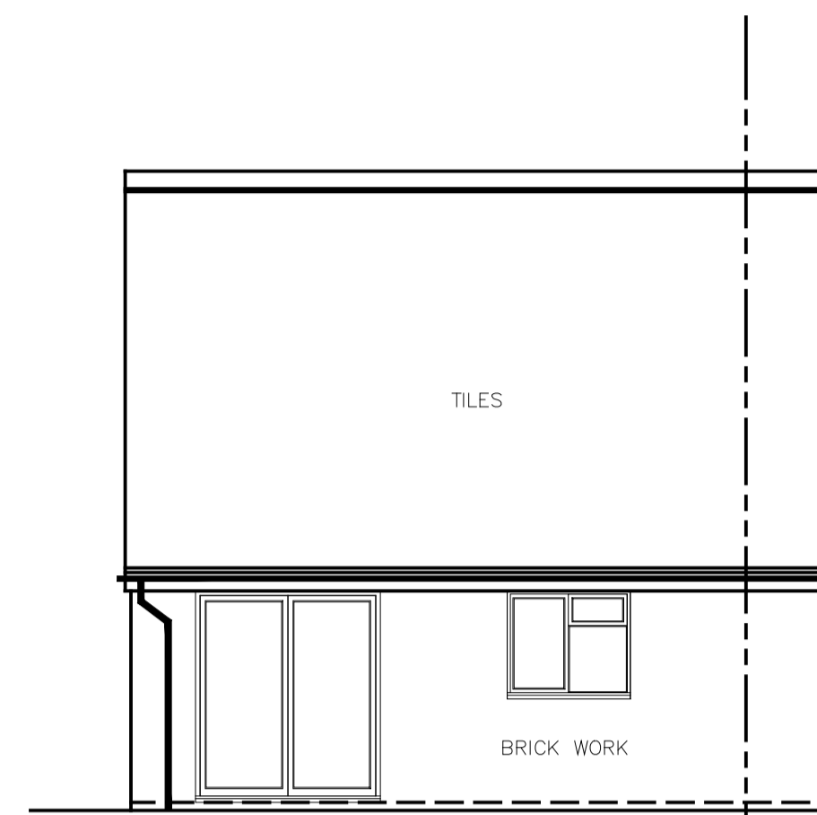
North Elevation Scale 1:100 0.0m 1.0m 2.0m 3.0m 4.0m 5.0m
