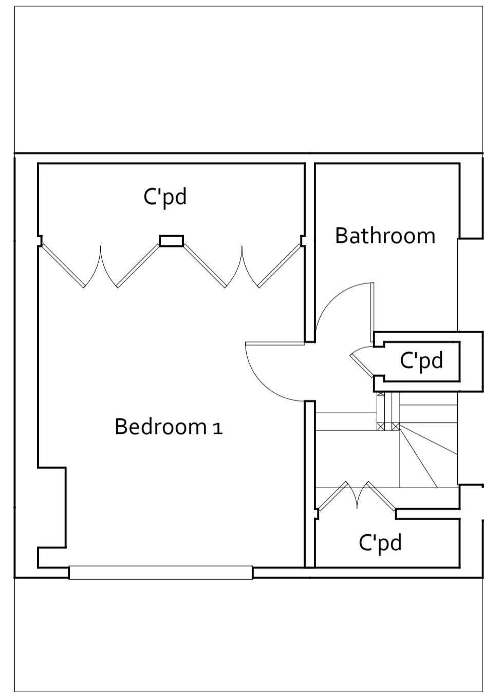
First Floor Scale 1:50 0.0m 1.0m 2.0m 3.0m 4.0m 5.0m
