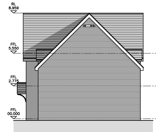
Right Elevation
