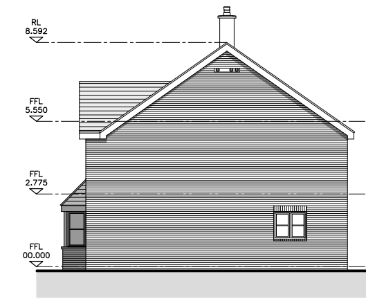
Right Elevation
