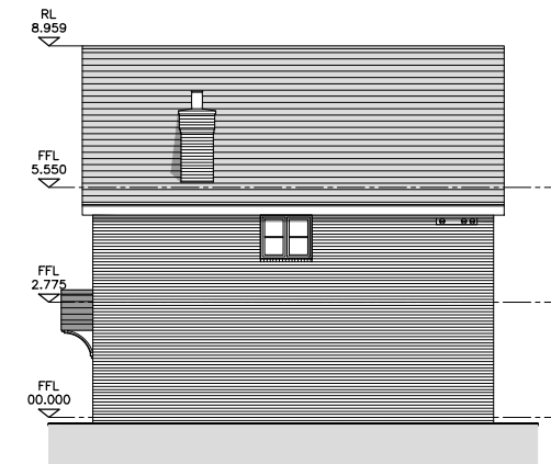
Right Elevation
