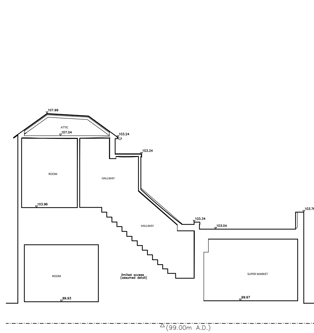
03 SECTION A-A 1:100
