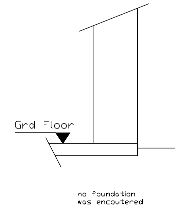
TP-3 (1:25)
