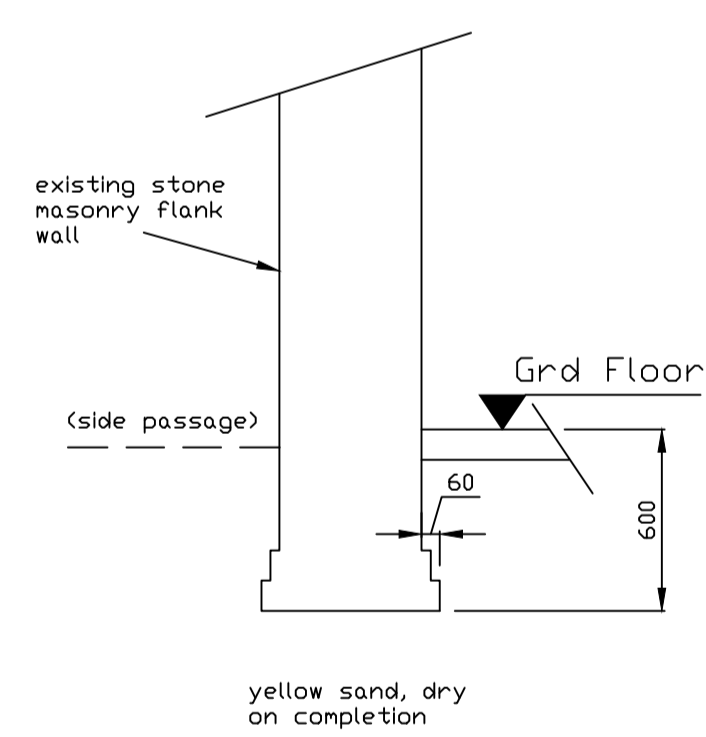
TP-2 (1:25)
