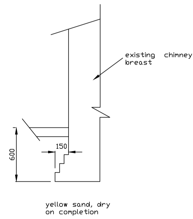
TP-2 (1:25)
