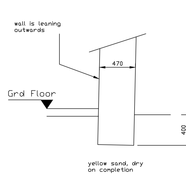
TP-1 (1:25)
