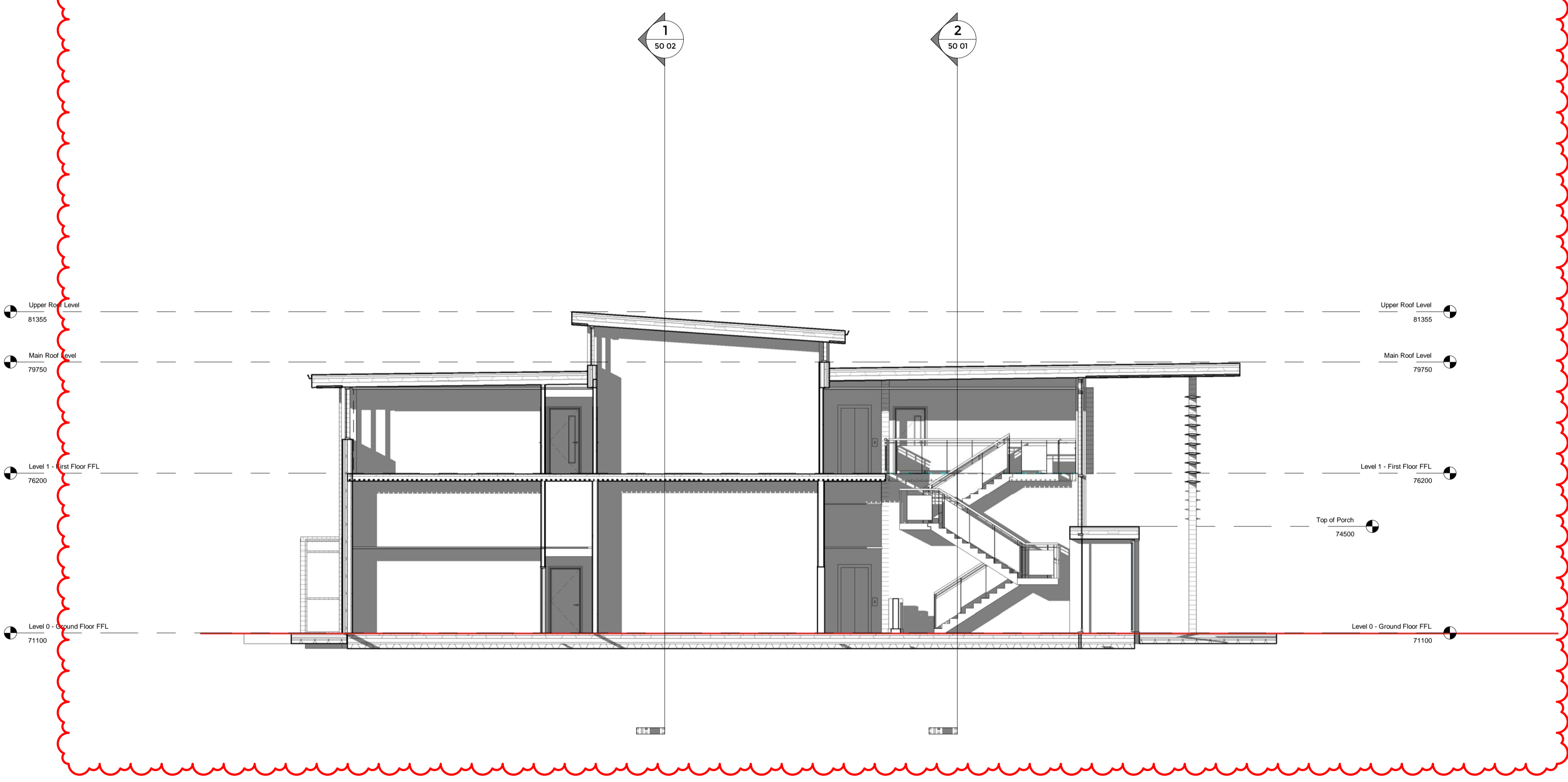
2 Section 4 1 : 100
